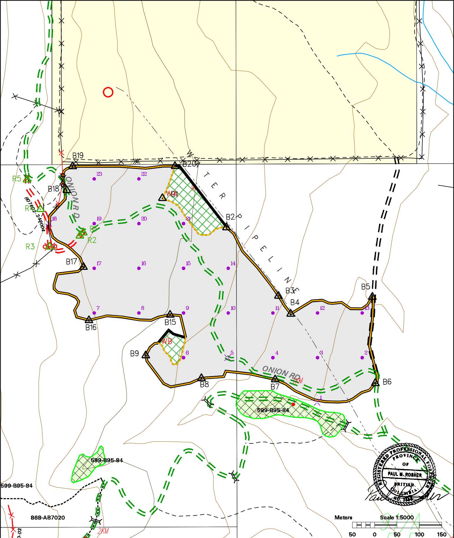
Site Plan 991-AB7028
